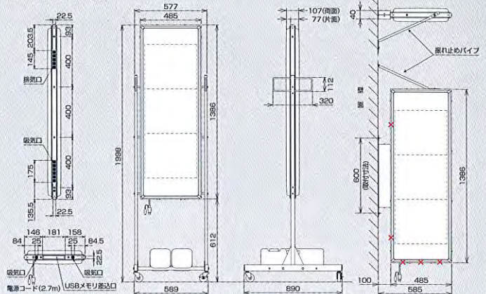
外観図 (単位/mm)
